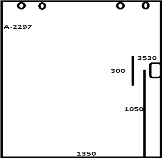
PORTA DE CORRER 8MM INCOLOR 1300X2260
